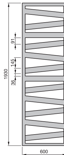
Pohled zepředu RB(C)-190-600
