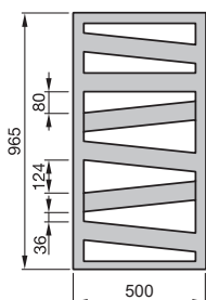
Pohled zepředu RB(C)-100-500
