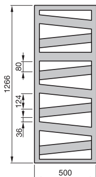
Pohled zepředu RB(C)-130-500
