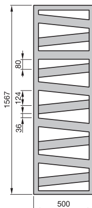
Pohled zepředu RB(C)-160-500
