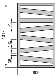
Pohled zepředu RB(C)-100-600 www.zehnder.cz
