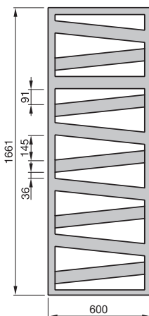
Pohled zepředu RB(C)-170-600
