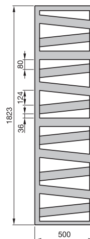
Pohled zepředu RB(C)-180-500
