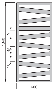
Pohled zepředu RB(C)-130-600
