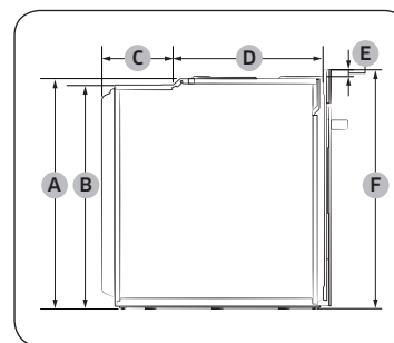
Rúra (mm)
