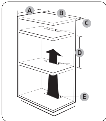
Vstavaná skrinka (mm)
