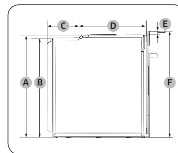
Trouba (mm)
