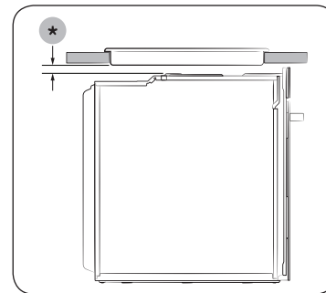
Inštalácia rúry
