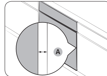
A sütő beszerelése
