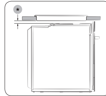
A sütő beszerelése
